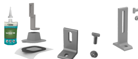
L-Foot & T-Foot
