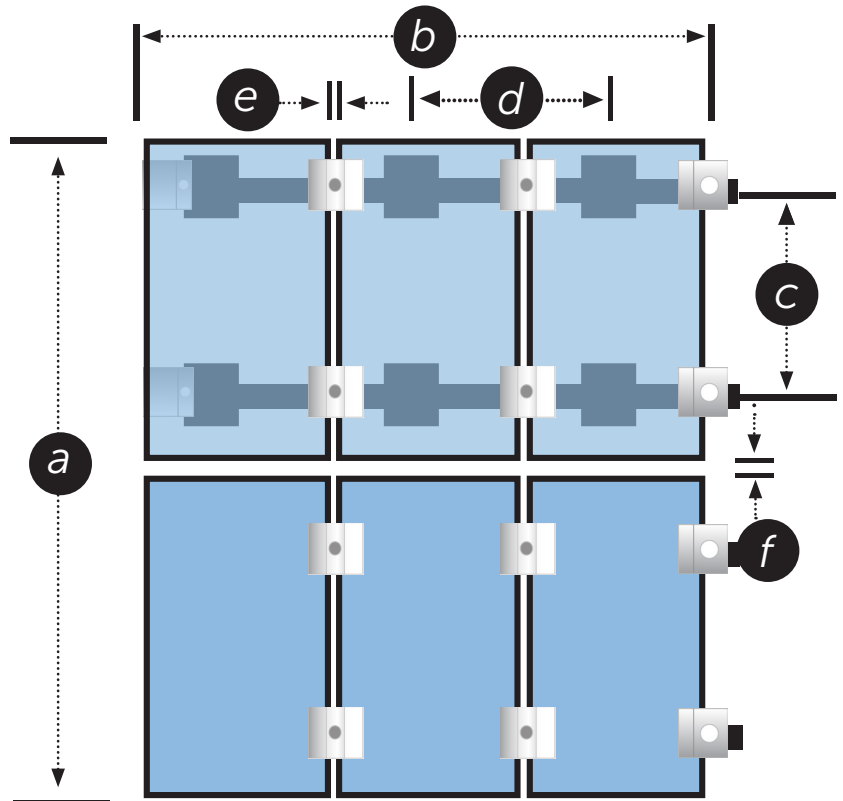
Image 4.1 Module Area
