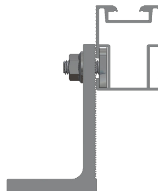
Image 2.4.12-2 L-foot / Rail / T-bolt
